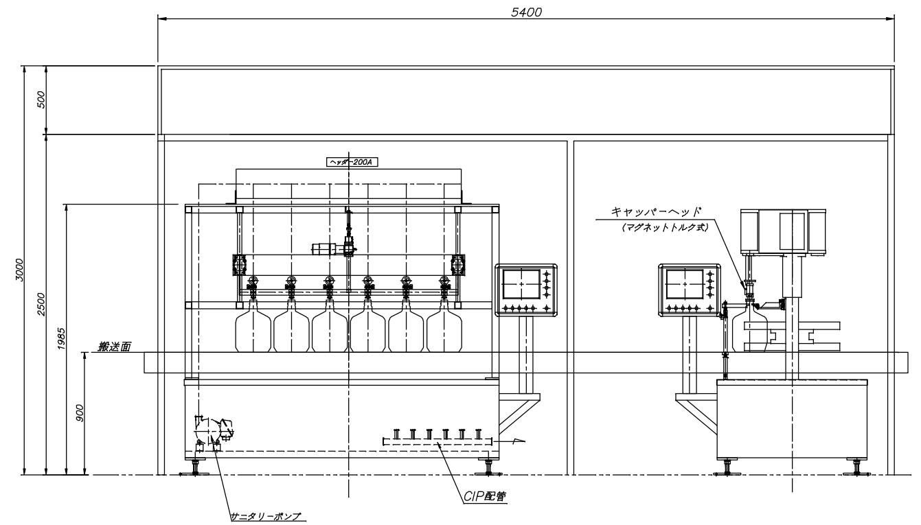
A 矢視図
